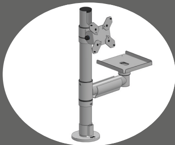
Art. Nr. 1027D Standrohr 500mm inkl. - VESA 75/100 Halterung - Seitenarm für Druckerplatte (200 oder 300mm) - Druckerplatte (produktspezifisch)
