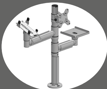
Art. Nr. 1027E Standrohr 600mm inkl. - VESA 75/100 Halterung - Seitenarm für Druckerplatte (200 oder 300mm) - Druckerplatte (produktspezifisch) - Seitenarm für EC-Cash (200 oder 300mm) - Halterung für EC-Cash (produktspezifisch)
